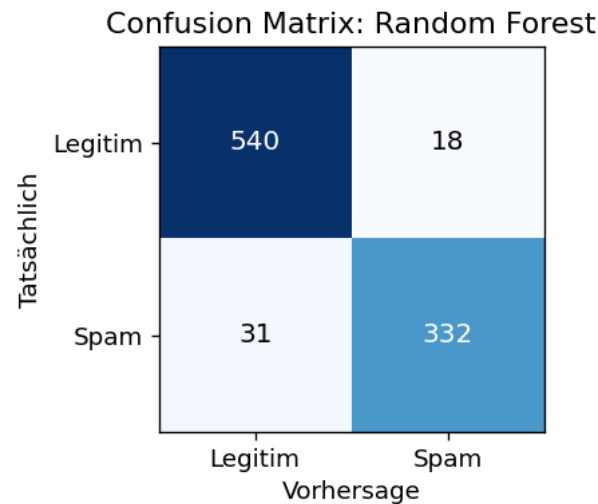
Abb. 7: Confusion-Matrix des Random Forest (Schwelle 0,5).
